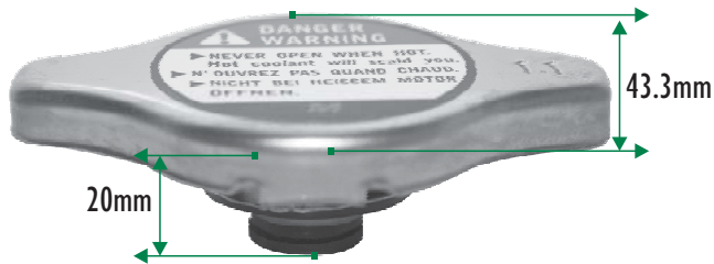
Tapón de 16 Libras
