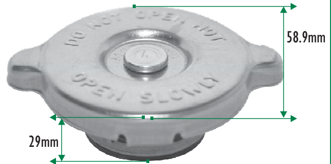
Tapón de 4 Libras
