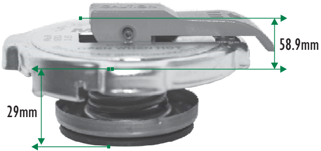
Tapón de 13 Libras con Palanca de Seguridad
