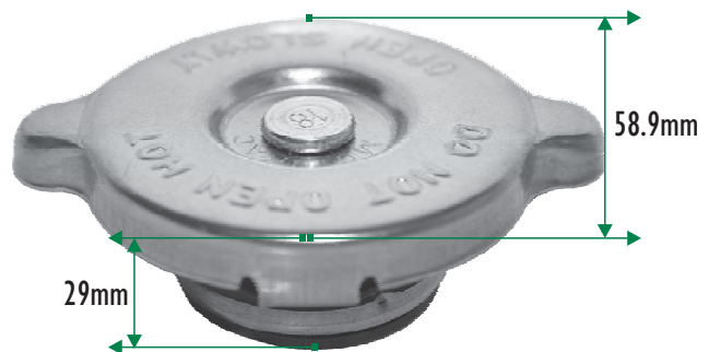
Tapón de 18 Libras
