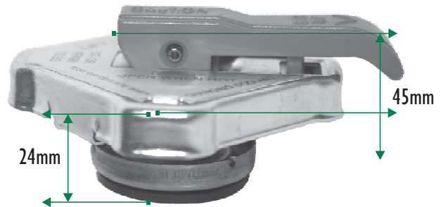
Tapón de 13 Libras con Palanca de Seguridad
