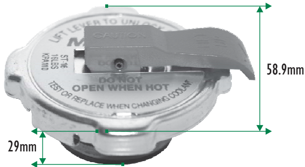
Tapón de 16 Libras con Palanca de Seguridad
