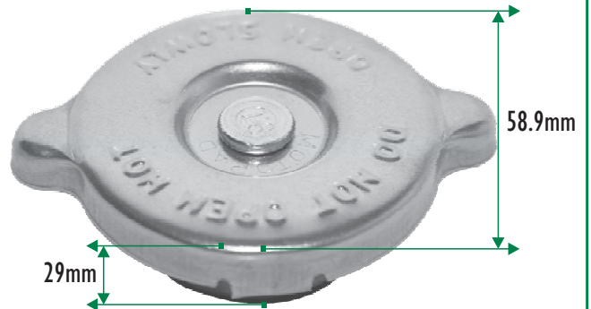
Tapón de 9 Libras
