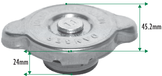
Tapón de 16 Libras
