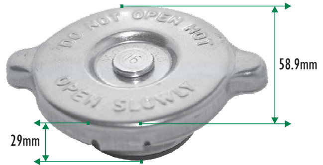
Tapón de 16 Libras
