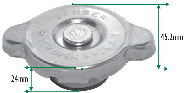
Tapón de 13 Libras
