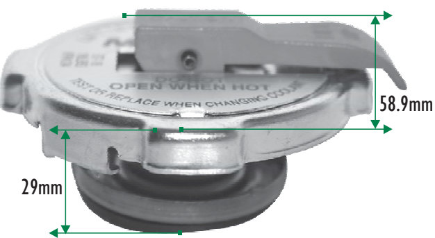
Tapón de 18 Libras con Palanca de Seguridad
