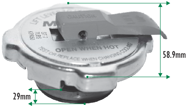
Tapón de 7 Libras con Palanca de Seguridad
