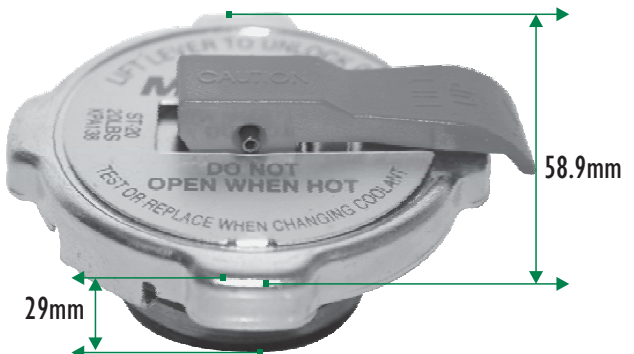
Tapón de 20 Libras con Palanca de Seguridad
